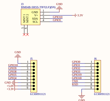
GPIO
